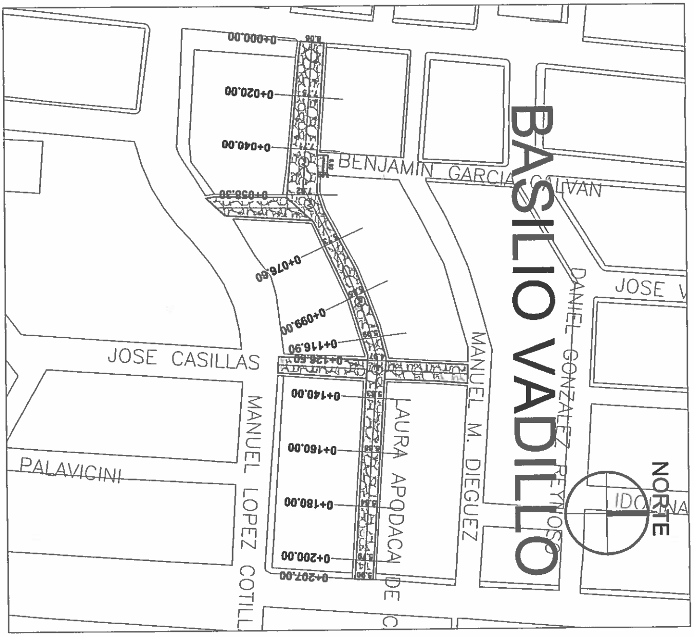
SECCIONES DE VALIDADES CON EMPEDRADO EN CAMA DE JALECILLO
