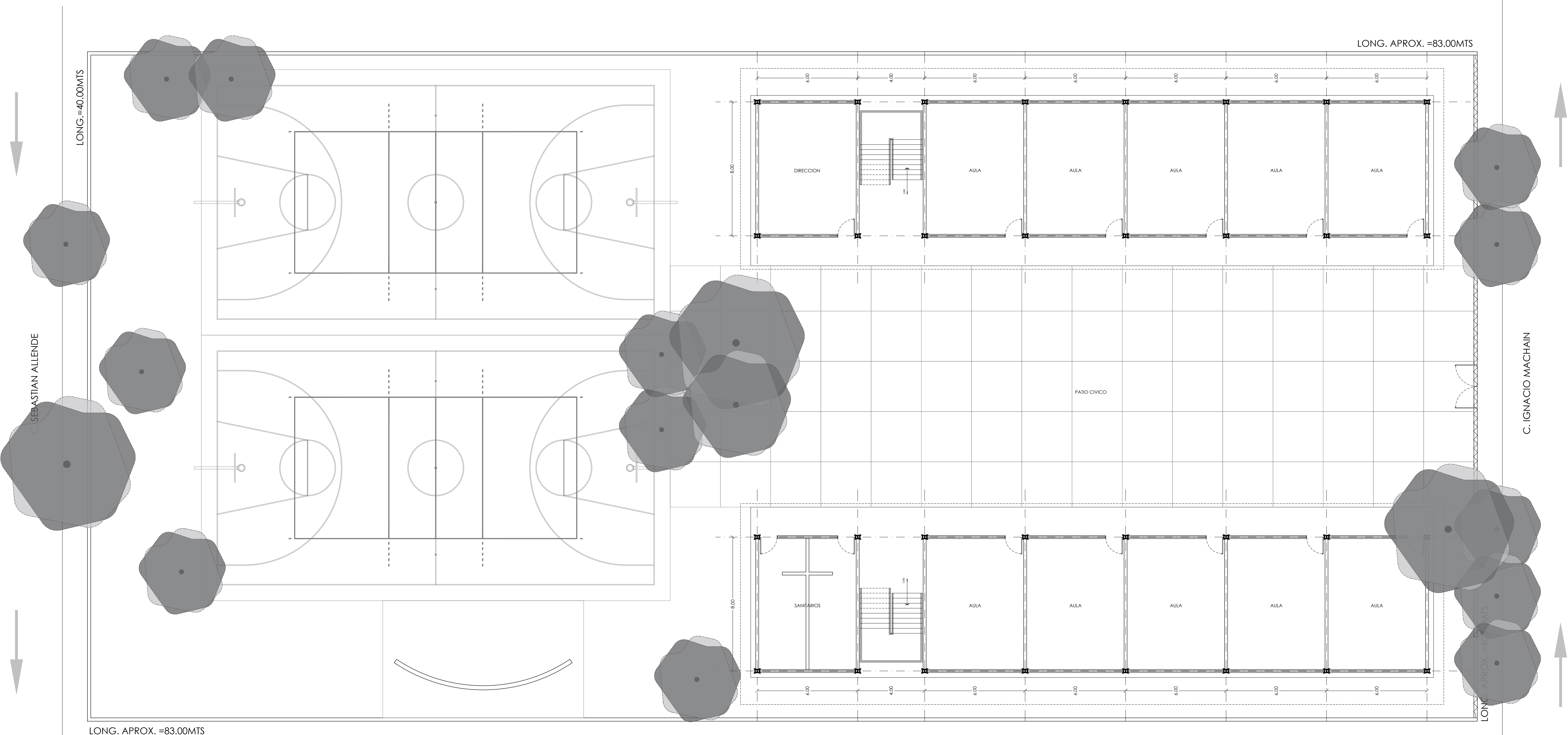
P. ARQUITECTONICA ESTADO ACTUAL 1:125
