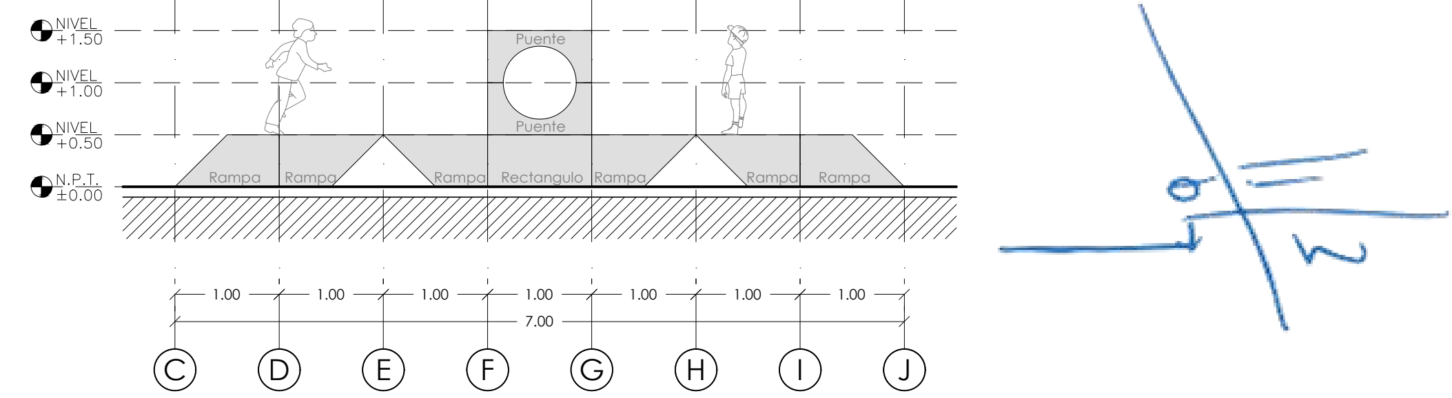
4 Alzado Juego 2 Esc. 1:50
