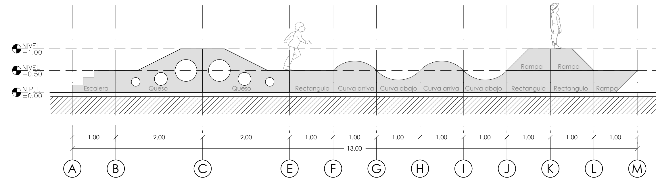
3 Alzado Juego 1 Esc. 1:50
