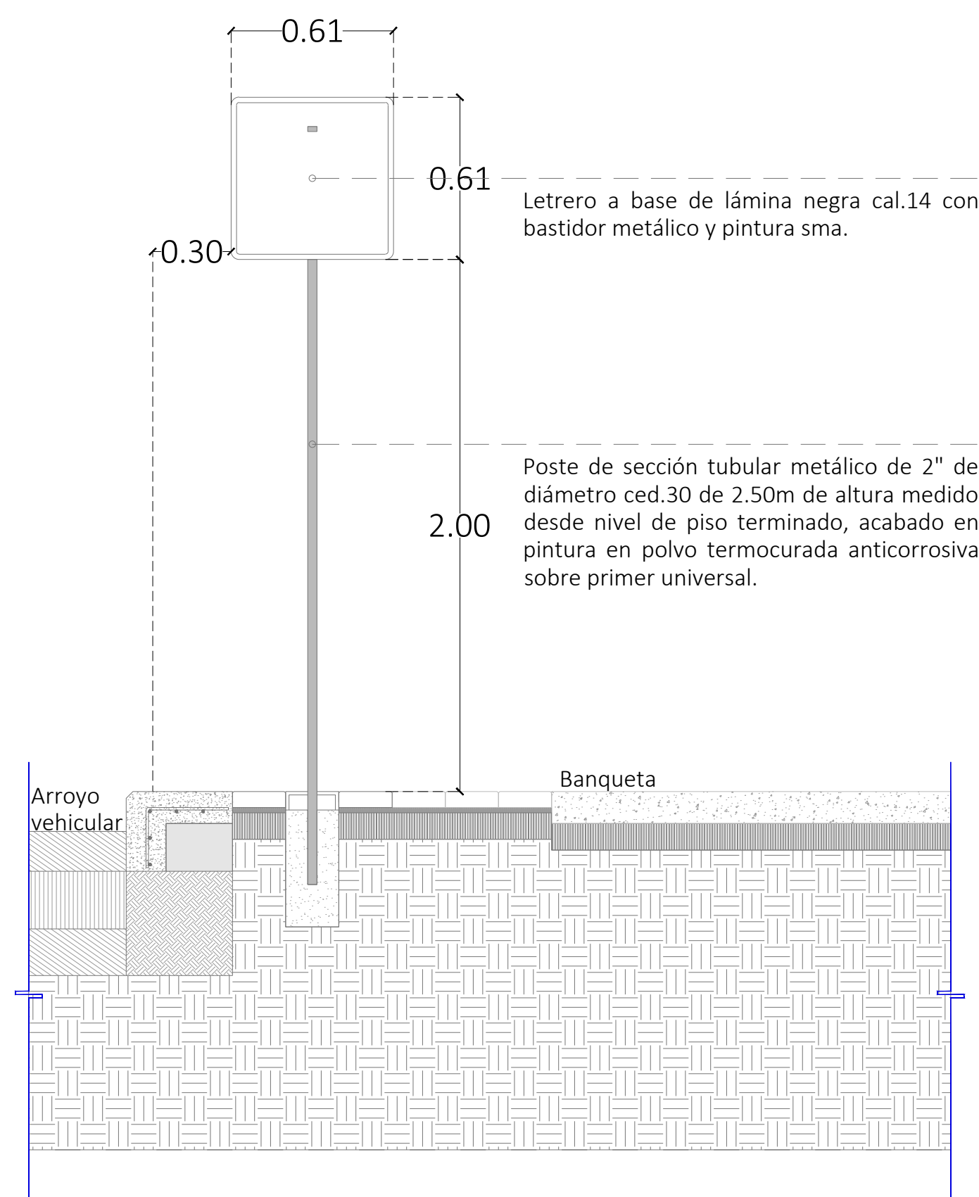
DETALLES DE SEÑALÉTICA VERTICAL ESC. 1:20
